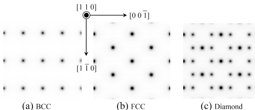
図 7.5 [1 1 0] 方向への電子密度の射影。(a) 体心立方格子, (b) 面心立方格子, (c) ダイヤモンド型格子について計算された
