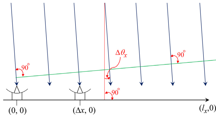
図 8.2 (0, 0) と (\Delta x, 0) の位置に並んだ 2 つのパラボラアンテナで構成される電波干渉計。右のアンテナは \Delta x 方向に可動であるとする
