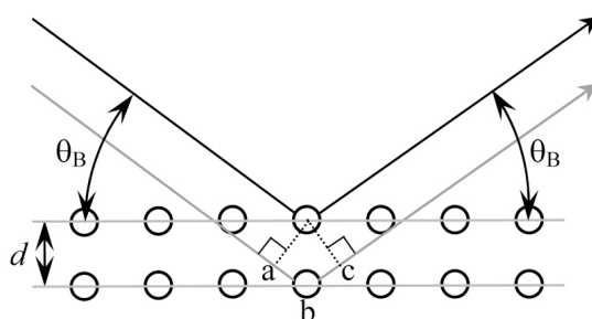
図 5.1 ブラッグの反射条件
