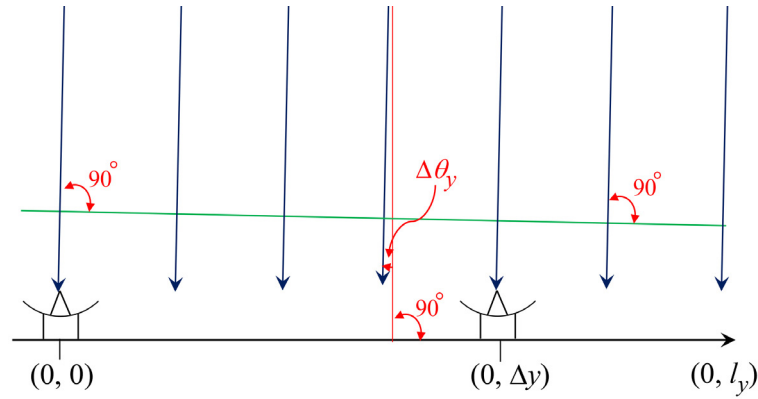
図 8.4 (0, 0) と (0, \Delta y) の位置に並んだ 2 つのパラボラアンテナで構成される電波干渉計。右のアンテナは \Delta y 方向に可動であるとする
