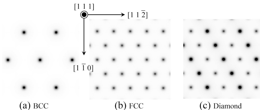
図7.4 [1 1 1] 方向への電子密度の射影。(a) 体心立方格子, (b) 面心立方格子, (c) ダイヤモンド型格子について計算された
