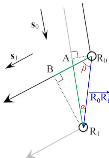
図 5.6 ラウエの反射条件
