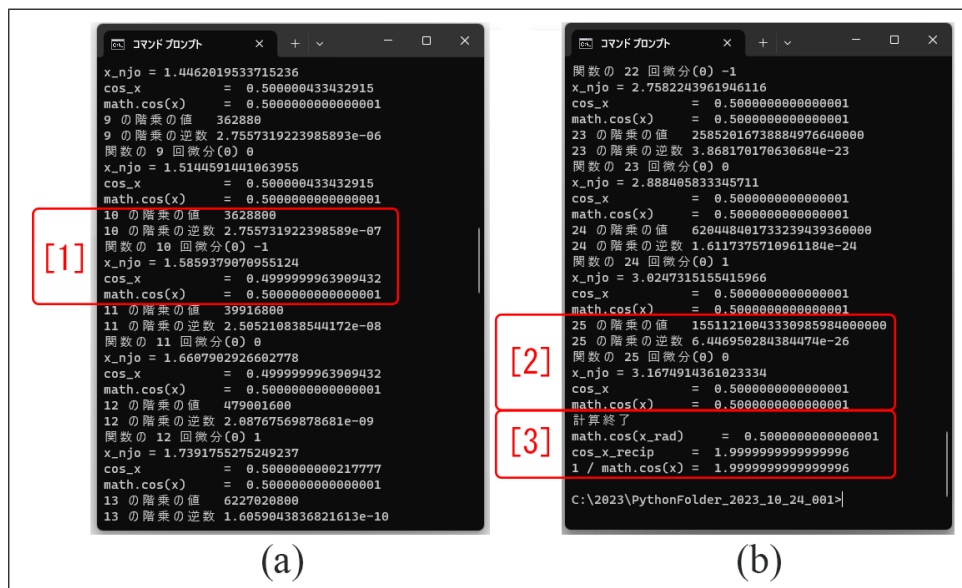
図 J.16 マクローリン展開による \cos(x) の計算プログラム
