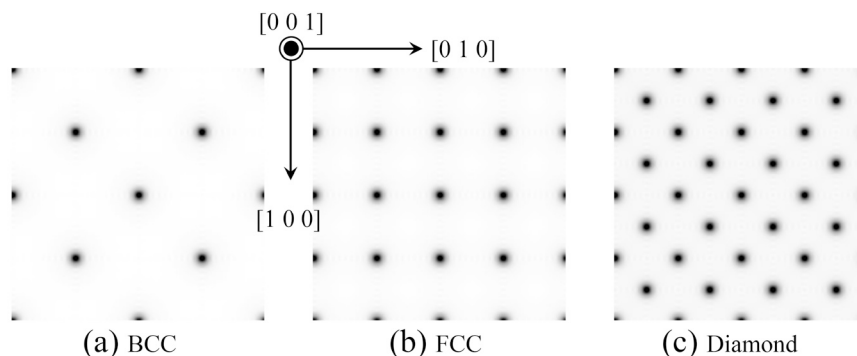
図 7.3 式 7.4a によって計算した x - y ( a - b ) 平面上への電子密度の射影 \rho(x, y) 。(a) 体心立方格子, (b) 面心立方格子, (c) ダイヤモンド型格子について計算された
