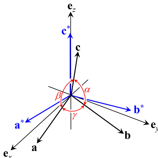
図 6.2 3次元の実格子基本並進ベクトル (黒) と逆格子基本ベクトル (青)。式 (6.45) によって式 (6.46), 式 (6.47) を満たすように逆格子基本ベクトルが定義されている
