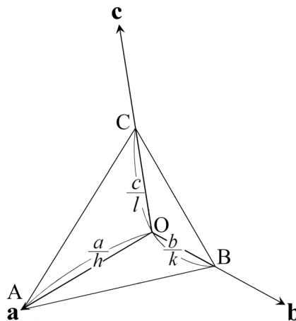
図 5.5 ミラーの作図法とミラー指数 [1]
