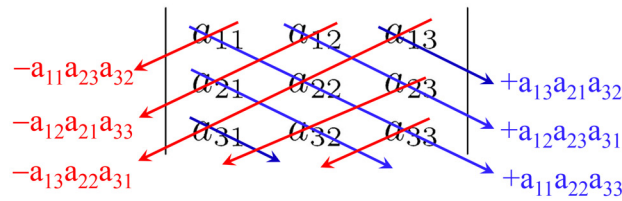
図 9.3 3 × 3 行列の行列式の計算 (サラスの公式, サラスの方法)。左上から右下へのかけ算 (青) はプラス, 右上から左下へのかけ算 (赤) はマイナスである
