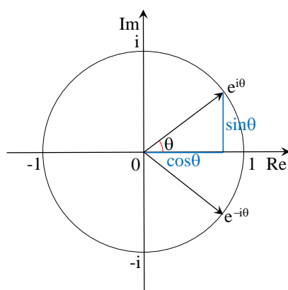
図 2.1 ガウス平面 (複素数平面)
