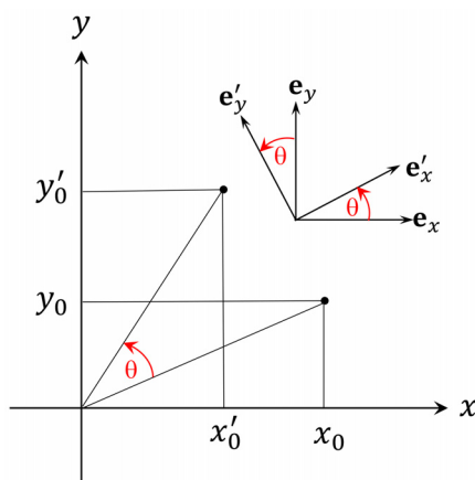
図 9.2 座標の回転
