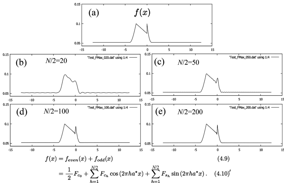
図 6.5 (a) もとの関数。式 (6.10) [p.63] で \infty の代わりに, (b) N/2 = 20 , (c) N/2 = 50 , (d) N/2 = 100 , (e) N/2 = 200 の有限な範囲でサンメーションを打ち切った級数による計算値
