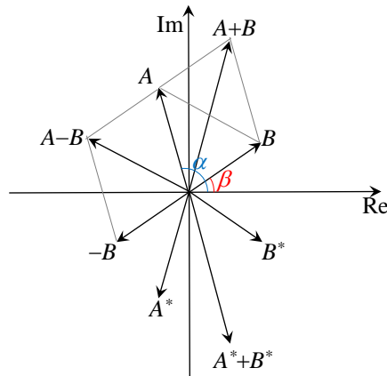
図 2.3 複素数の足し算と引き算は、2次元のベクトルと同様におこなわれる
