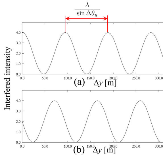
図 8.5 (a) (0, 0) の位置に固定されたアンテナと (0, \Delta y) の位置にあり \Delta y 可変のアンテナで構成される電波干渉計による干渉強度。(b) 固定されたアンテナが受信した電波の位相を \pi/2 遅らせたときの干渉強度
