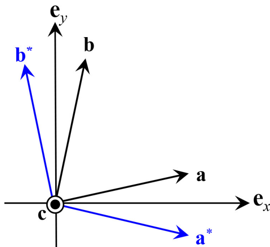
図 6.1 2次元の実格子基本並進ベクトル (黒) と逆格子基本ベクトル (青)。式 (6.33) によって式 (6.34) を満たすように, 逆格子基本ベクトルが定義されている
