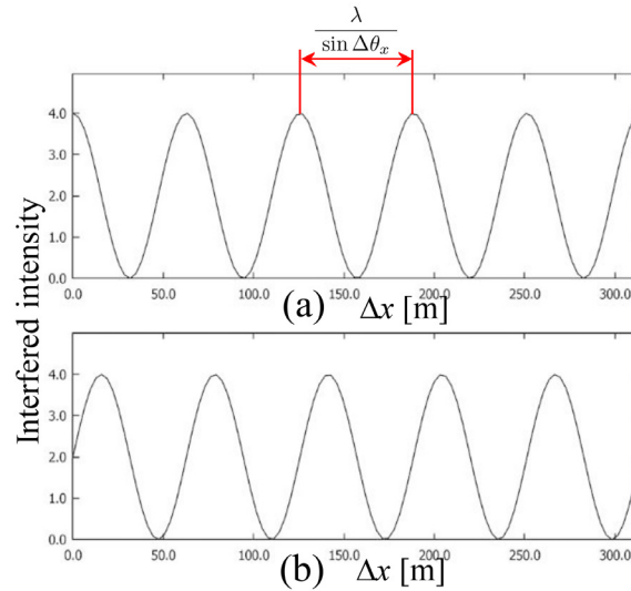
図 8.3 (a) (0, 0 の位置に) 固定されたアンテナと (\Delta x, 0) の位置にありに \Delta x が可変のアンテナで構成される電波干渉計による干渉強度。(b) 固定されたアンテナが受信した電波の位相を \pi/2 遅らせたときの干渉強度
