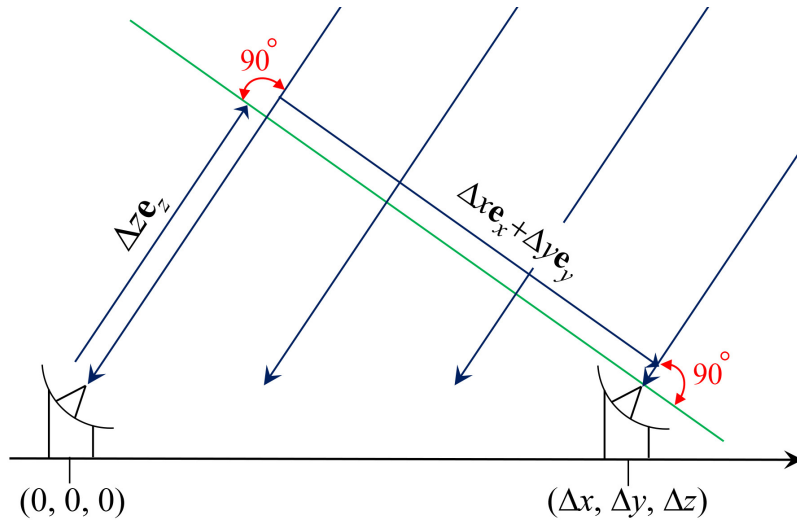
図 8.6 天体を追尾中のパラボラアンテナ
