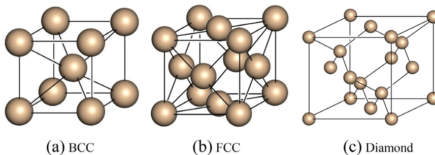
図 7.2 (a) 体心立方格子, (b) 面心立方格子, (c) ダイヤモンド型格子の原子配列
