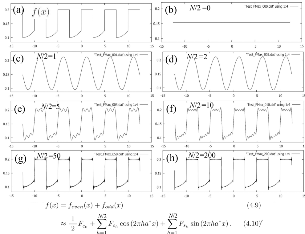
図 6.4 (a) もとの関数。式 (6.10) [p.63] で \infty の代わりに、(b) N/2 = 0 , (c) N/2 = 1 , (d) N/2 = 2 , (e) N/2 = 5 , (f) N/2 = 10 , (g) N/2 = 50 , (h) N/2 = 200 の有限な範囲でサンメーションを打ち切った級数による計算値
