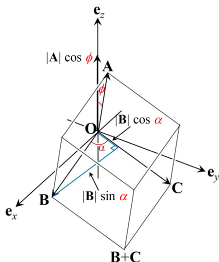
図 B.5 \mathbf{A} , \mathbf{B} , \mathbf{C} のスカラー三重積はこれらのベクトルを稜とする平行六面体の体積である。図 4.3 [p.39] の再掲
