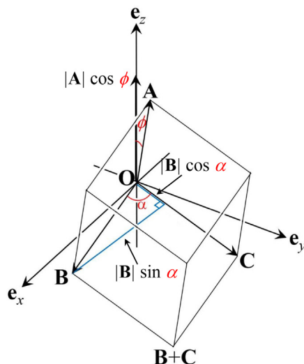
図 4.3 A, B, C のスカラー三重積はこれらのベクトルを稜とする平行 6 面体の体積である
