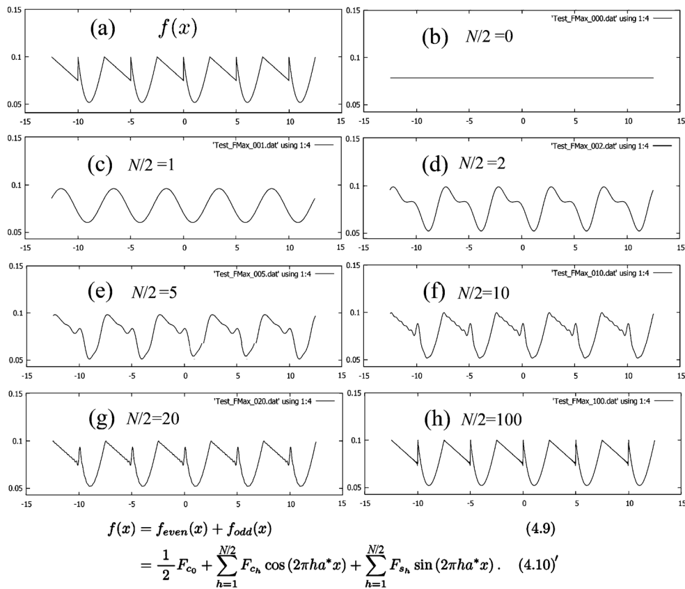
図6.3 (a) もとの関数。式(6.10) [p.63] で \infty の代わりに, (b) N/2 = 0 , (c) N/2 = 1 , (d) N/2 = 2 , (e) N/2 = 5 , (f) N/2 = 10 , (g) N/2 = 20 , (h) N/2 = 100 の有限な範囲でサンメーションを打ち切った級数による計算値
