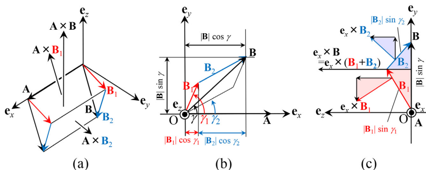
図 4.2 \mathbf{A} と \mathbf{B} 内積と外積, および分配法則。(b) と (c) はそれぞれ, (a) を \mathbf{e}_z と \mathbf{e}_x の方向から見た図
