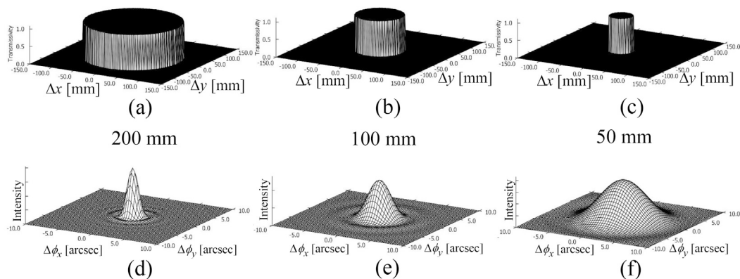
図 8.1 望遠鏡の対物レンズ (対物鏡) の口径 [(a) 200 mm, (b) 100 mm, (c) 50 mm] と光の回折角 (光軸からのズレ角) の関係。光の波長を 500nm であると仮定している。(d), (e), (f) は、それぞれ (a), (b), (c) を高速フーリエ変換することにより得られている。レンズないしは反射鏡は焦点付近に天体の像を作るが、(d), (e), (f) はその像のボケに相当する
