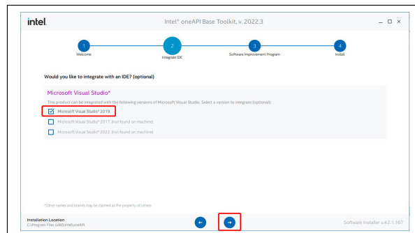
図 I.36 「Microsoft Visual Studio 2019」にチェックが入っていることを確認して右向き矢印をクリック
