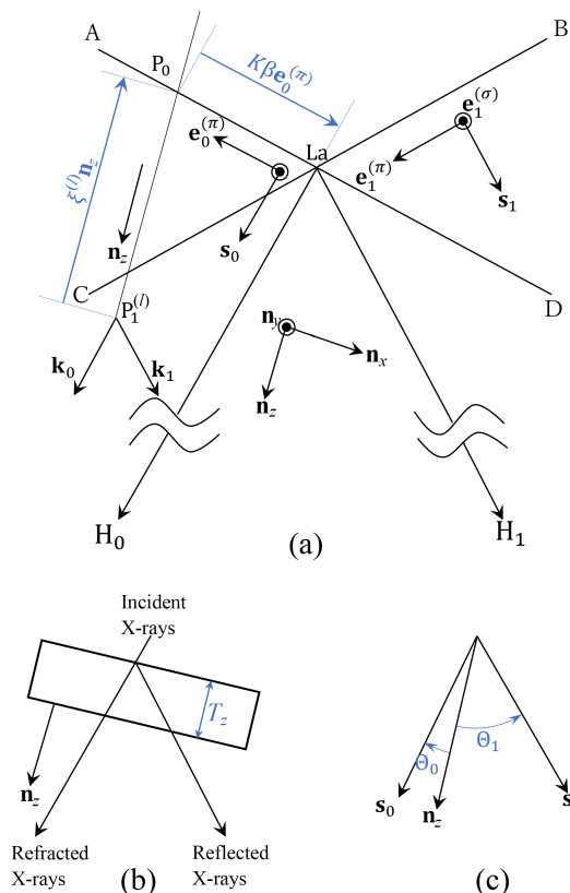
図 K.3 ラウエケース
