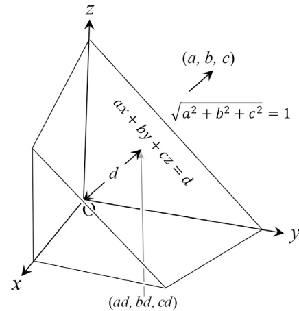
図 B.3 x - y - z 次元空間の平面
