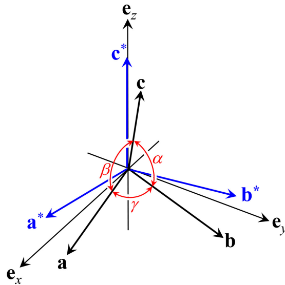
図 4.2 3次元の実格子基本並進ベクトル (黒) と逆格子基本ベクトル (青)。式 (4.45) によって式 (4.46), 式 (4.47) を満たすように逆格子基本ベクトルが定義されている
