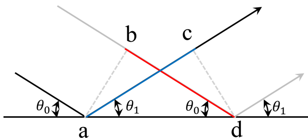
図 8.3 鏡に対する光の入射角 ( \theta_0 ) と反射角 ( \theta_1 ) が同じになる理由
