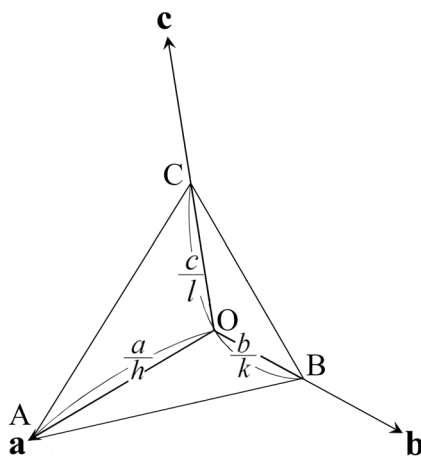
図 8.5 ミラーの作図法とミラー指数 [1]
