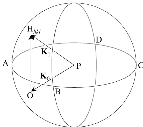
図 8.4 エバルト球
