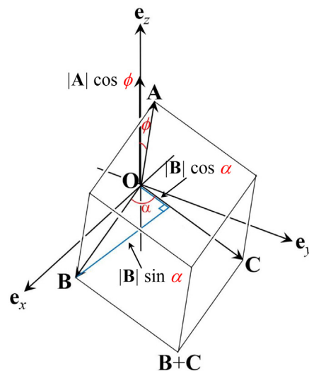
図 5.3 A, B, C のスカラー三重積はこれらのベクトルを稜とする平行 6 面体の体積である
