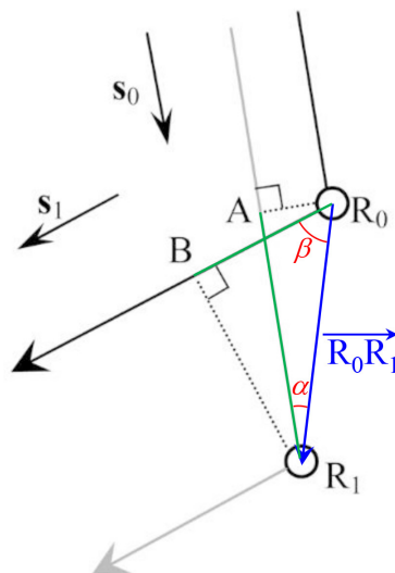
図 8.6 ラウエの反射条件
