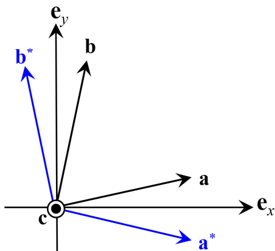
図 4.1 2次元の実格子基本並進ベクトル (黒) と逆格子基本ベクトル (青)。式 (4.33) によって式 (4.34) を満たすように, 逆格子基本ベクトルが定義されている
