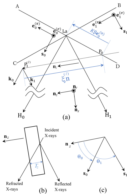
図 K.4 ブラッグケース
